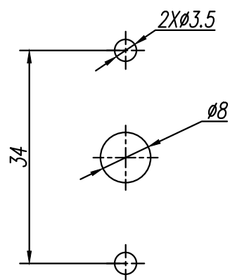
HZ5-10/1.7 M05 组合开关外形尺寸图
