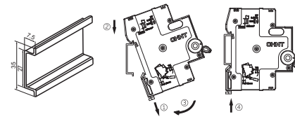
图3 安装示意
