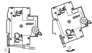
图4 拆卸示意
