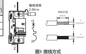
图5 接线方式
