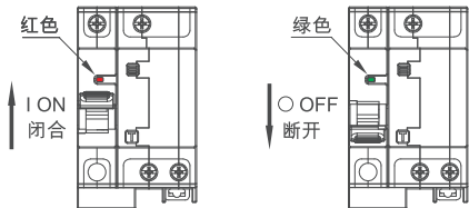
图2 闭合、断开状态指示
