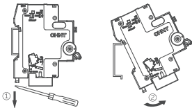
图4 拆卸示意图
