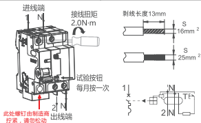
图5 接线示意图
