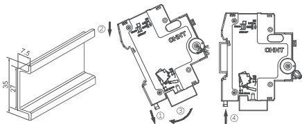
图3 安装示意图
