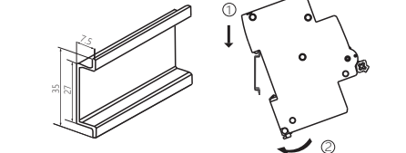
图3 安装示意
