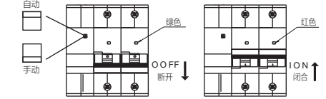
图2 产品手动、自动状态, 闭合、断开状态指示
