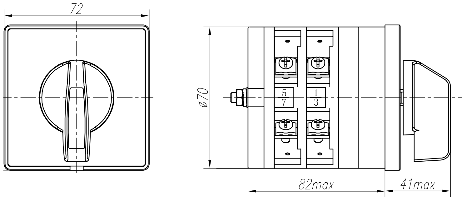
LW5D-16/2 万能转换开关外形尺寸图
