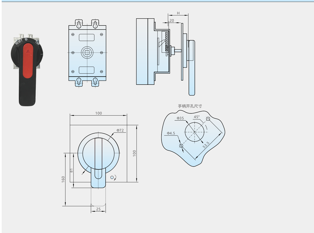
操作机构外形及安装尺寸图
