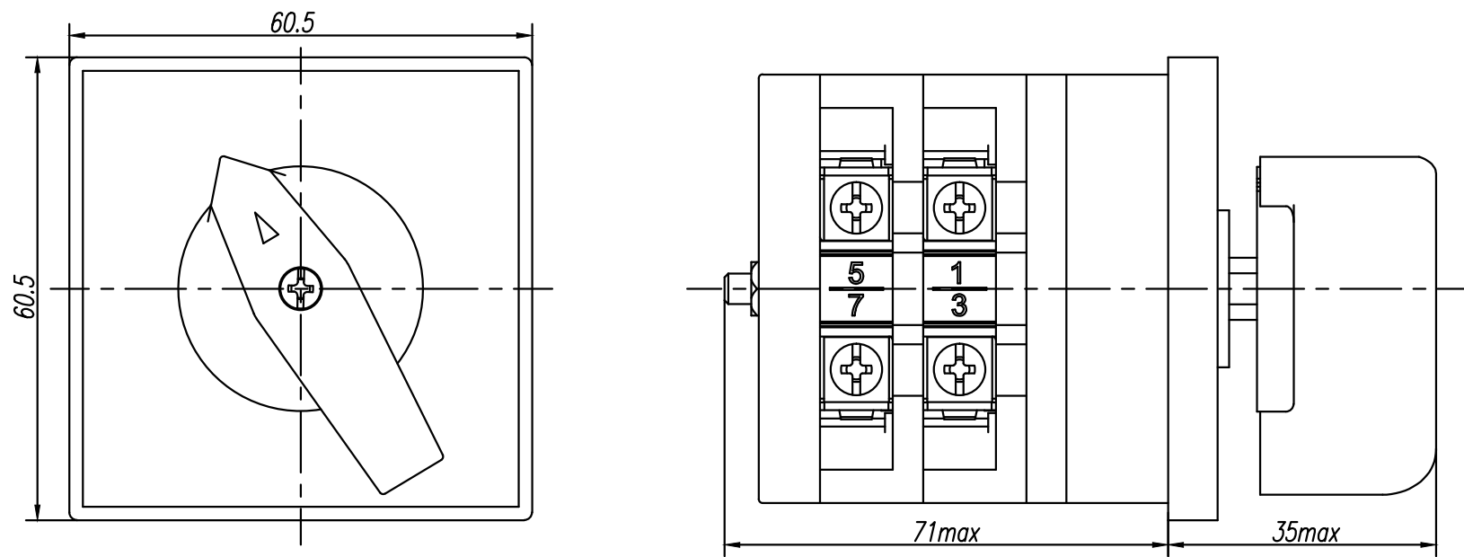
HZ5-20/4 L03 组合开关外形尺寸图
